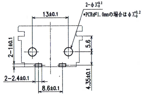
基板取付穴参考寸法
