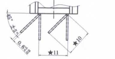
端子形状C
